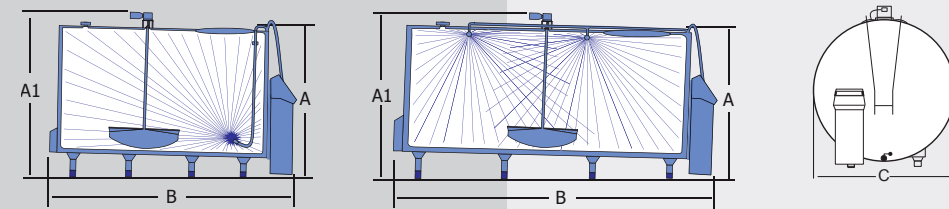
Mallista O 2000 ja P 8000 alkaen säiliöt varustettu suihkusuuttimilla (irroittettava suutinputki).
